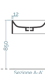
Sezione A-A'
